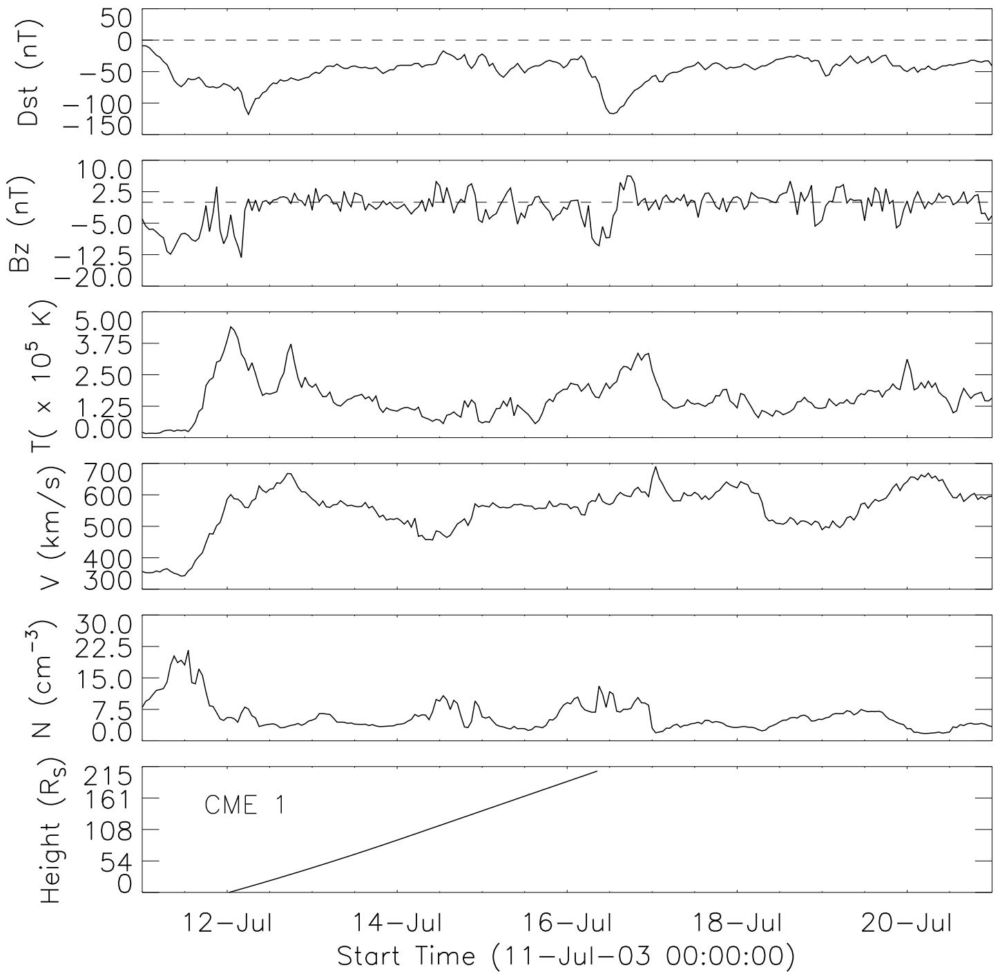
CME1: 2003/07/12 00:30:05, -----, V= 331, Sc=1.00, W=118
